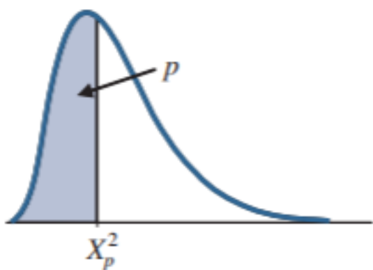
Tavola C.2 Quantili della distribuzione chi-quadrato.
